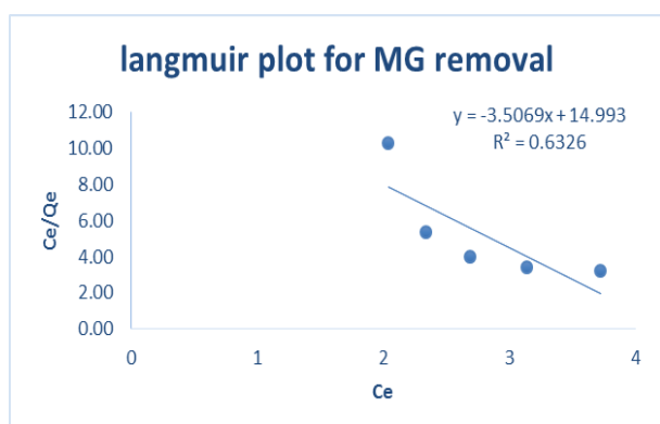
Fig. 5: Langmuir Equilibrium.
