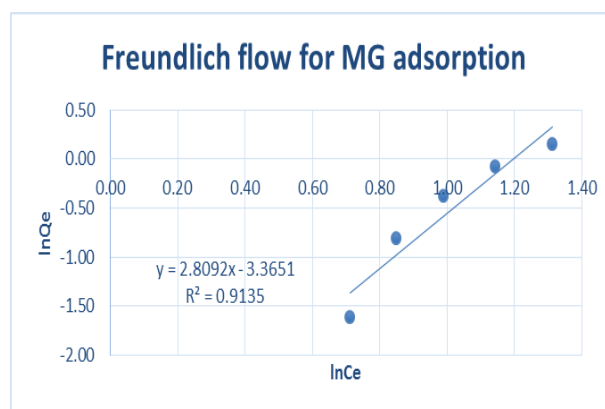
Fig. 6: Freundlich Equilibrium.
