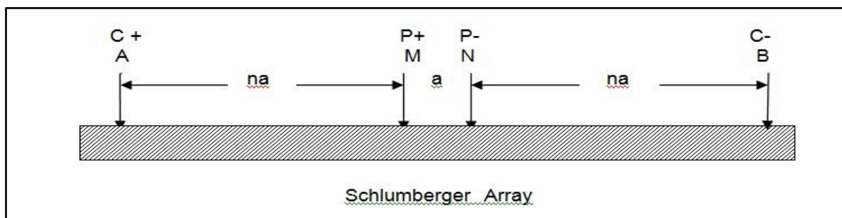
Fig. 2.0. Schlumberger Array
